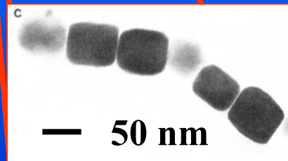
Cubic
